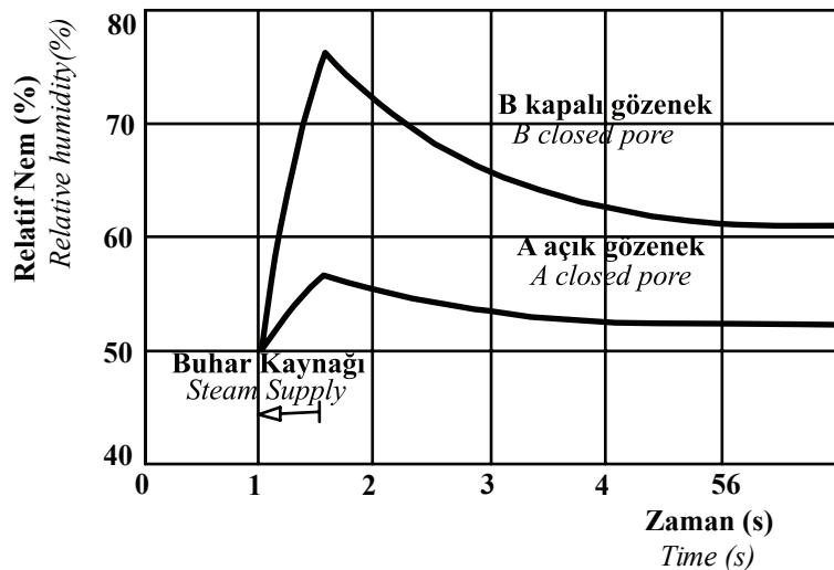
Şekil 3.9. Bağıl Nemin Duvar Yüzey Özelliğine Göre Değişmesi [39] Figure 3.9. Change in Relative Moisture According to Wall Surface Characteristic [39]
