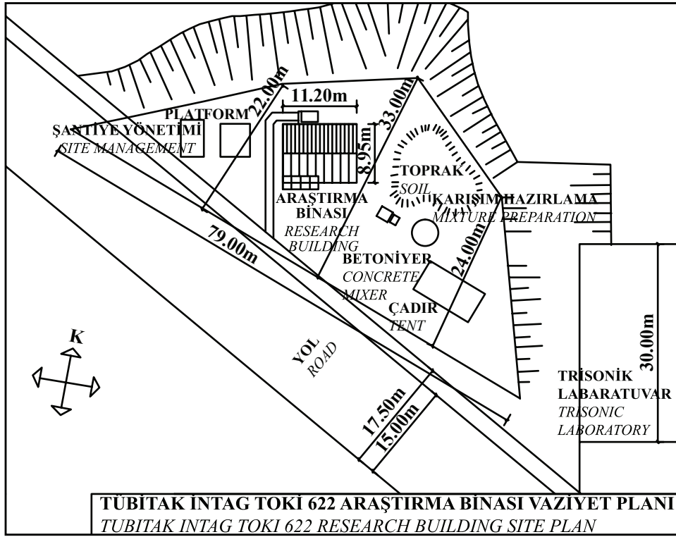
Şekil 3.4. İTAK TOKİ 622 Kerpiç Yapı Projesi Vaziyet Planı (Rektörlük Tahsisi)
