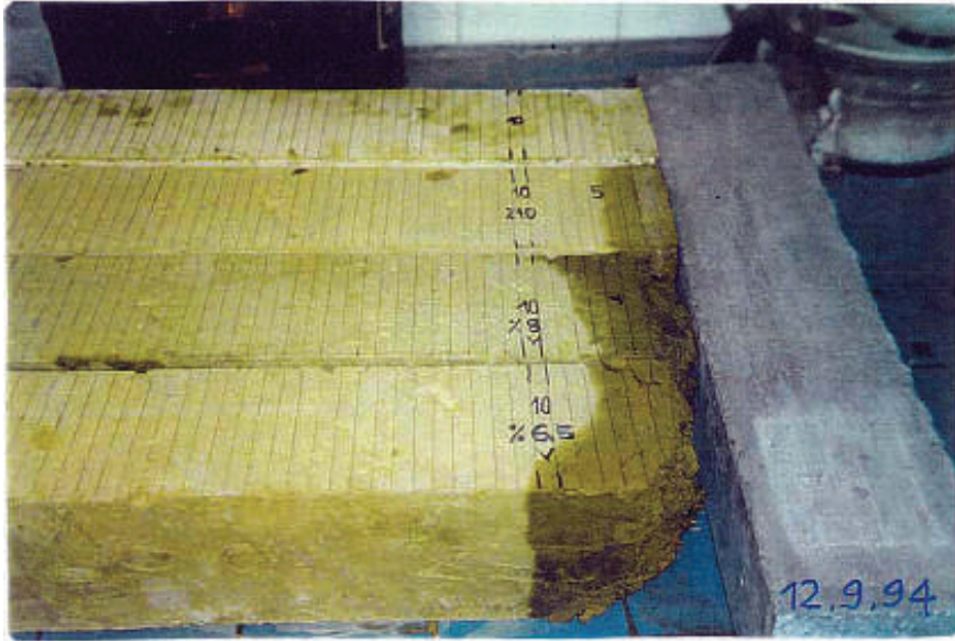
Resim 2.3. %10 Katkılı Alçı İle Hazırlanan Numunelerde 24 Saat Sonunda Suyun Yükselme Miktarları
