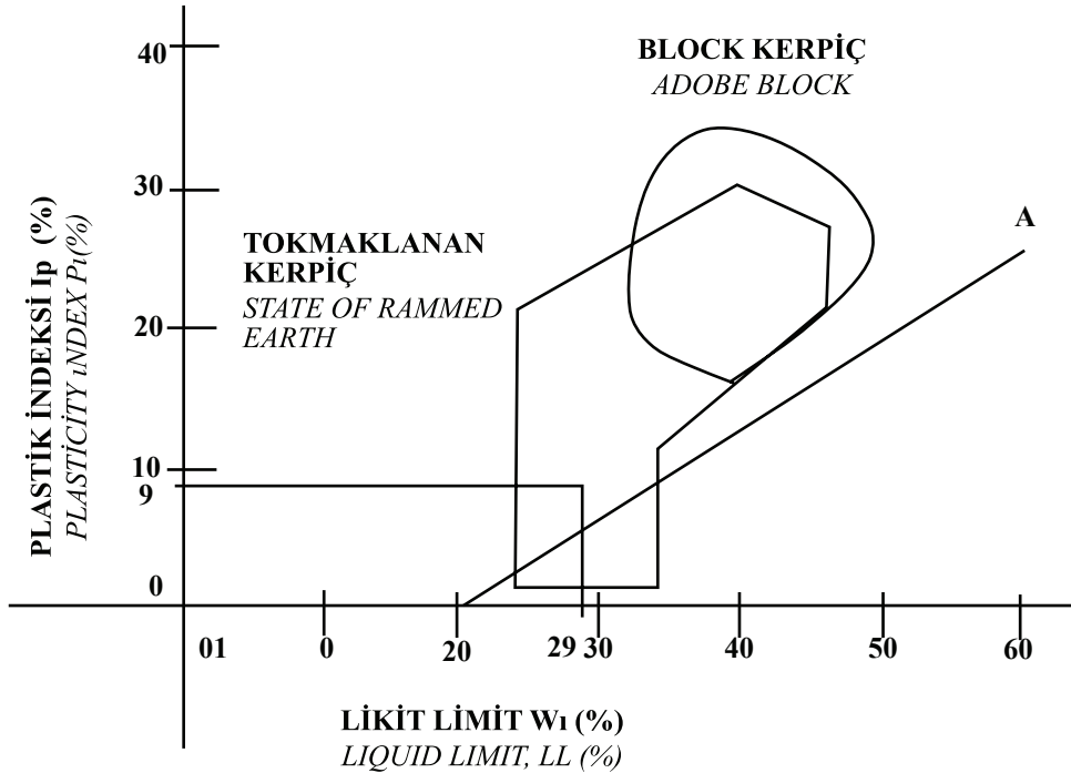
Şekil 2.4. Plastisite Diyagramı [19]
