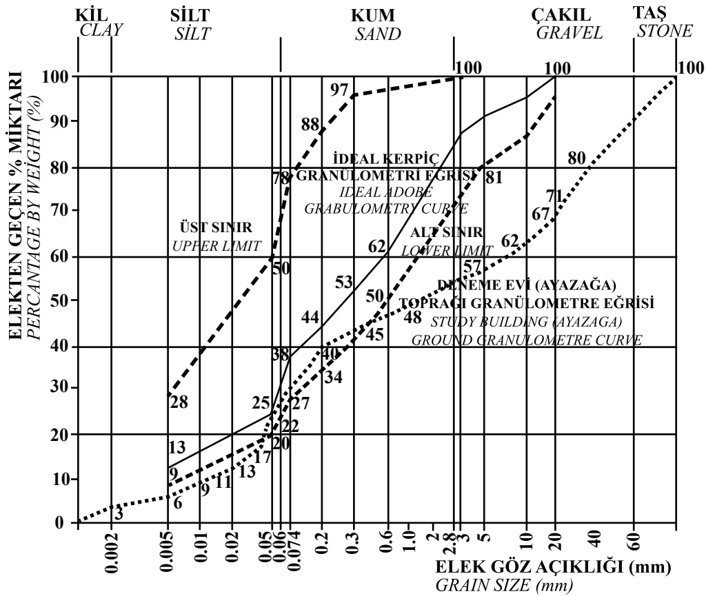
Şekil 2.3. Araştırmada Kullanılan Ayazağa Toprağının Granülometrik Eğrisi.
