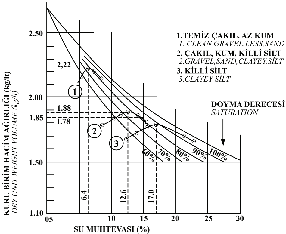
Şekil 2.5. Proctor Eğrileri [21]
