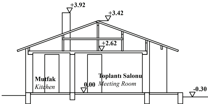
Şekil 3.10 İNTAG TOKİ 622 Alçılı Kerpiç Yapı Projesi Figure 3.10 İNTAG TOKİ 622 Gypsum Stabilized Adobe Building Project
