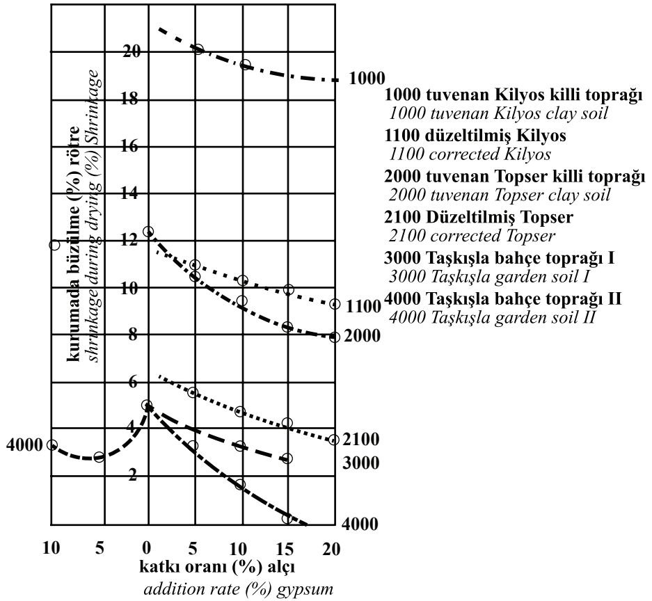
Şekil 2.6. Farklı Toprak Türlerinin Alçı-Kireç Oranlarına Bağlı Olarak Rötreye Değişimleri [11] Figure 2.6. Shrinkage Changes of Different Soil Types According to Gypsum- Lime Rates [11]
