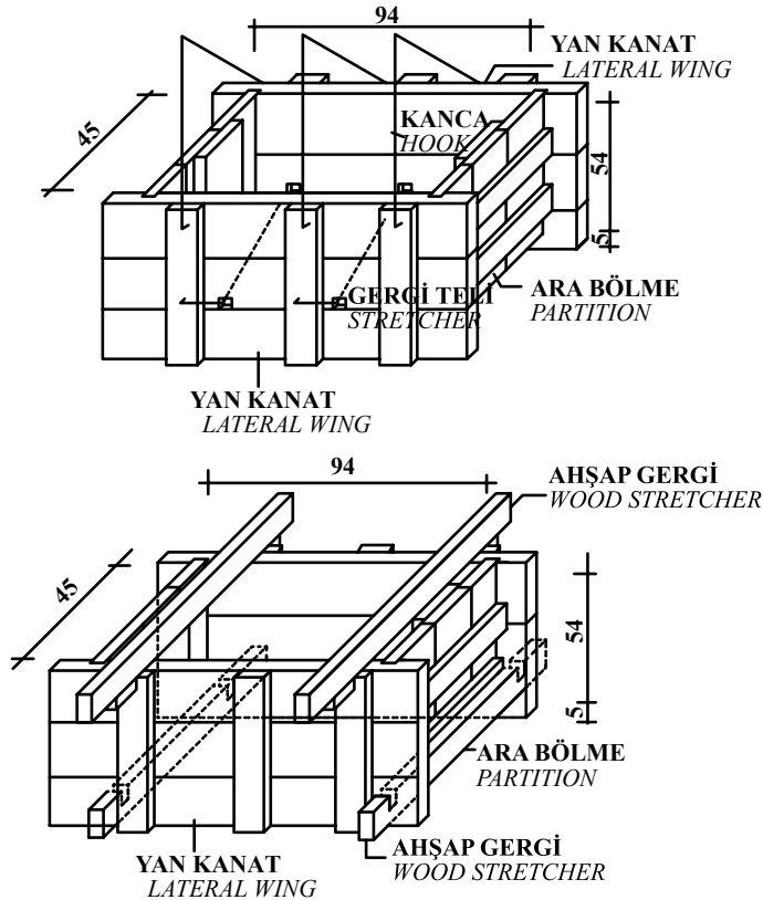
Şekil 3.6. Münferit Yerinde Döküm Kalıbı
