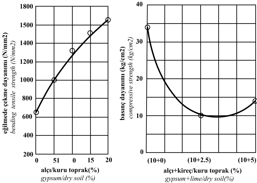
Şekil 2.9. Bahçe Toprağından Üretilmiş Numunelerin (A) Alçı Katkı Oranına Bağlı Eğilmede Çekme Dayanımı Değişimi (B) %10 Alçı Katkılı Bahçe Toprağına Katılan Kireç Oranına Bağlı Olarak Basınç Dayanım Değişimi [12]
