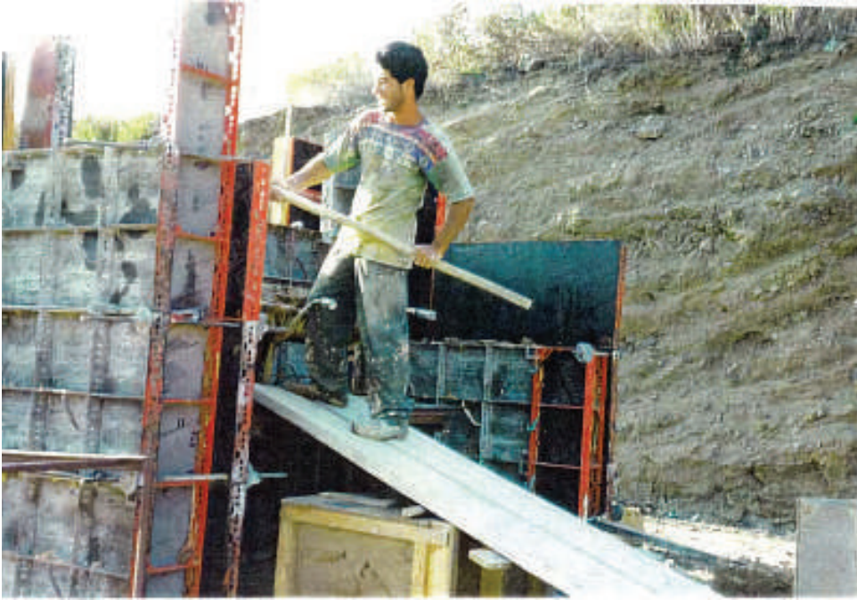
Resim 3.9. Karışımın El Arabasından Kalıplara Boşaltılması Picture 3.9. Discharge of the Mixture from Handcarts into Moulds
