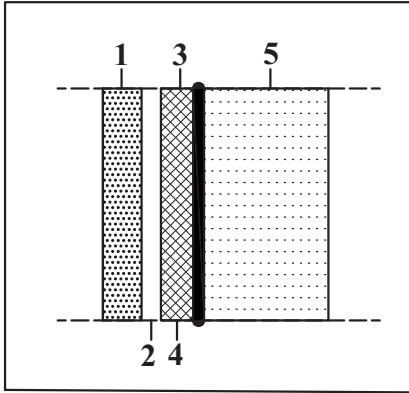
Şekil 3.8. Malzemenin Yangında Davranış Sınıfı [38] Figure 3.8. Behavior Class of the Material During Fire [38]
