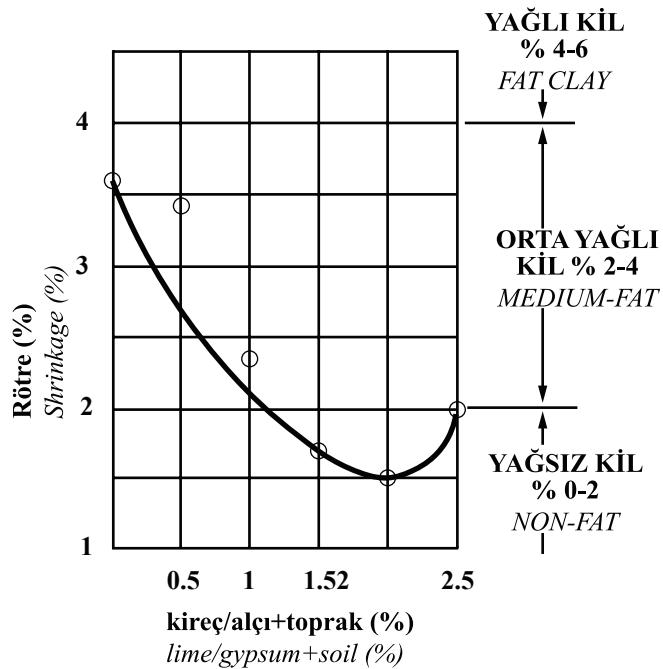
Şekil 2.10. %10 Katkılı Alçı İle Hazırlanan Numunelerde Kireç Katkısı Oranına Bağlı Olarak Rötre Değişimi.
