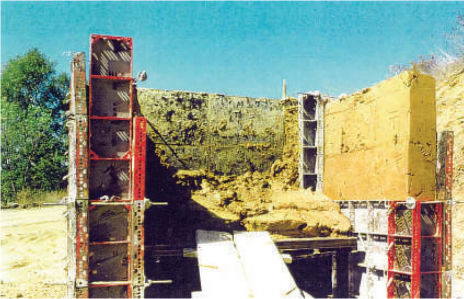
Resim 3.14. Alçının Priz Süresi Dışında Uygulanan Rövibrasyon Metodunun Sonucu Picture 3.14. The Result of Rovibration Method Applied out of Gypsum's Setting Time
